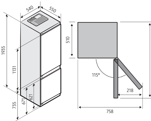
Le misure si intendono in mm
